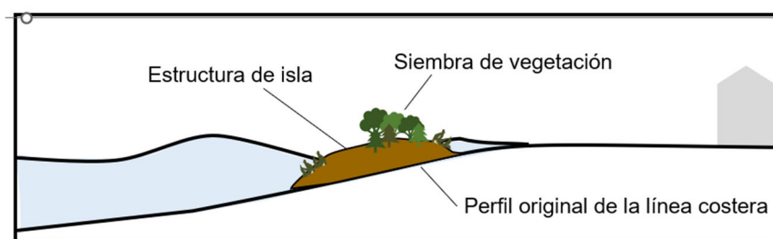
Gráfica 11. Boceto conceptual de una estructura de isla para aumentar la protección ante inundaciones y reducir la erosión
