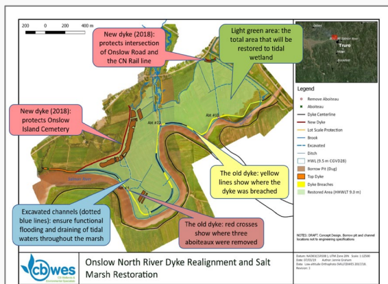
Gráfica 8. Diseño del sitio del proyecto río Onslow-North River
