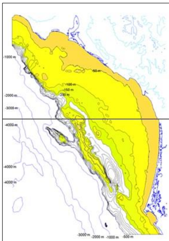
Mapa 5 Batimetría general de la región del Golfo de Ulloa
