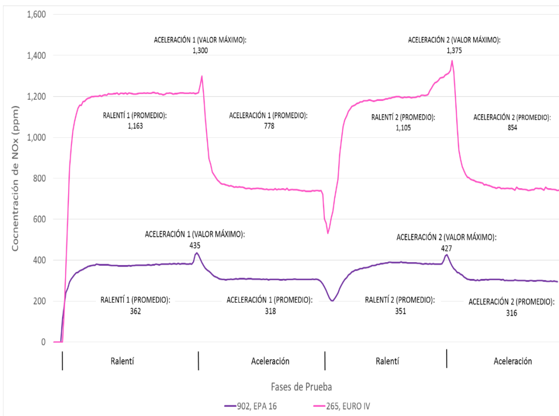
Figura 3 Comparativa de emisión de emisiones de NOx de un vehículo EPA 16 y un vehículo EURO IV
