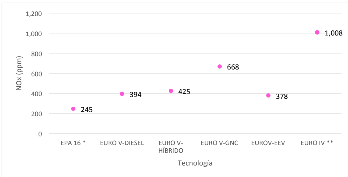
Figura 4 Emisión de NOx (promedio)
