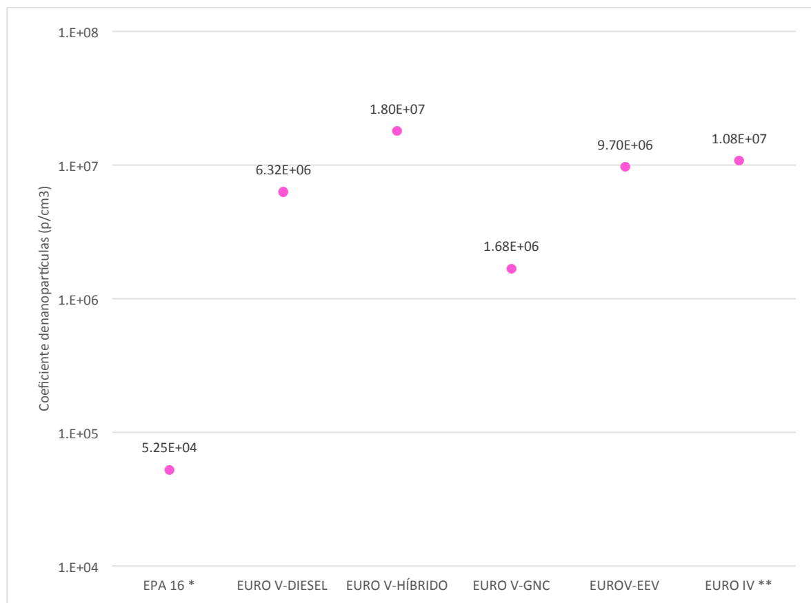
Figura 6 .Emisión de número de partículas
