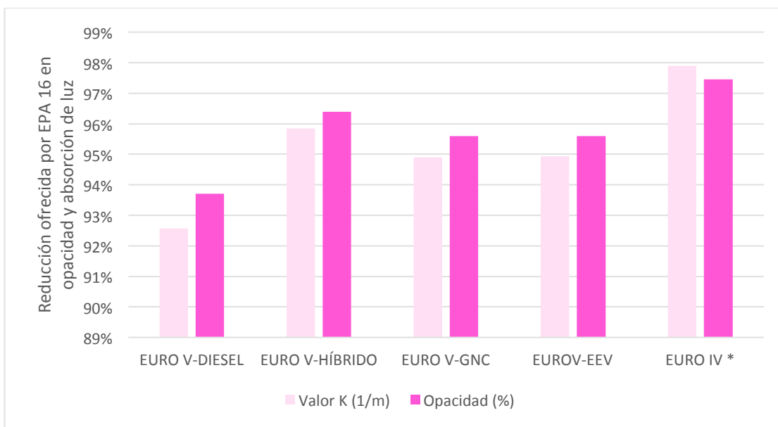
Figura 5. Reducción en opacidad y absorción de luz ofrecido por los vehículos EPA 16 (en promedio) comparados a los vehículos de EURO V-Diésel, EURO V-Híbrido, EURO V-GNC, EURO V-EEV y EURO IV.
