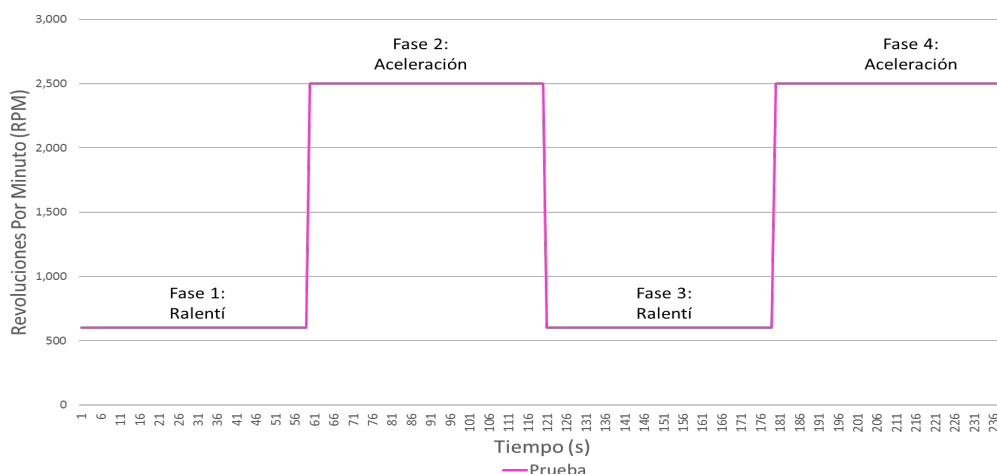
Figura 2. Representación de las cuatro fases de cada prueba
