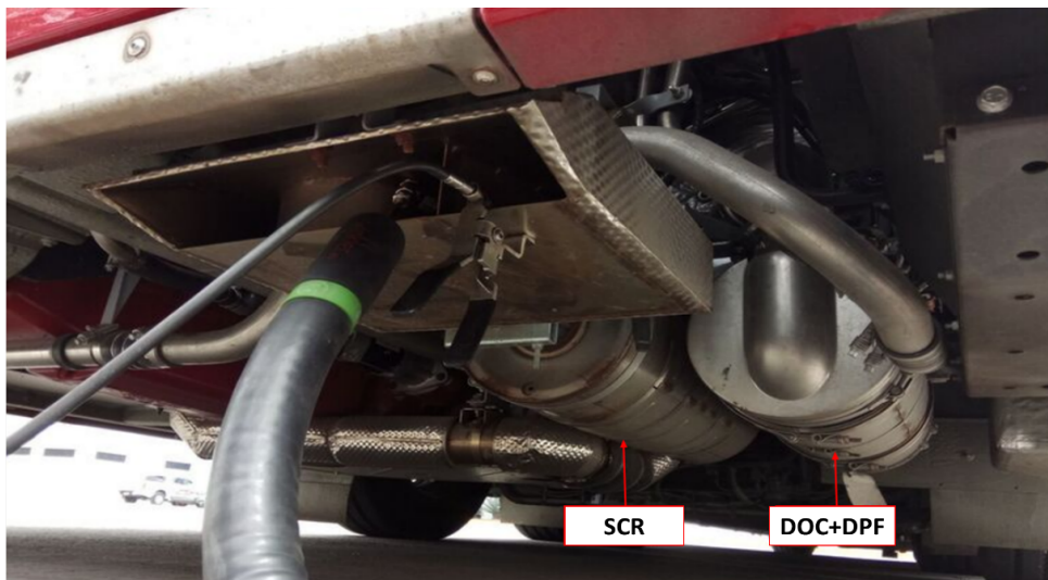
Figura 1. Distribución de los sistemas de tratamiento de gases de escape (SCR-DPF) de los vehículos Enviro 500
