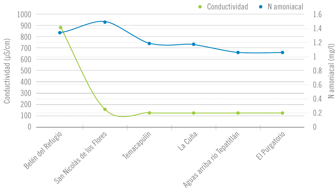
Figura 23. Conductividad y nitrógeno amoniacal en el río Verde 527
