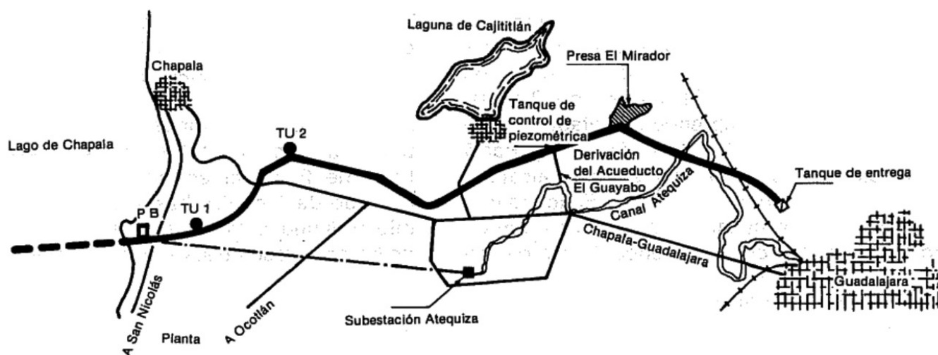
Figura 7. Acueducto Chapala-Guadalajara y estructuras principales 304
